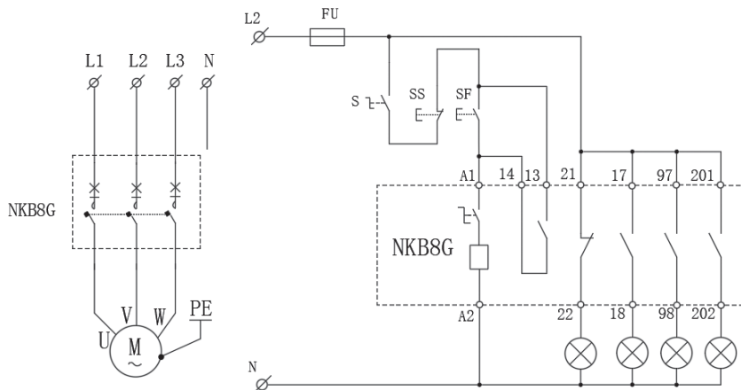
Рис. 3. Базовая схема управления для NKB8G
