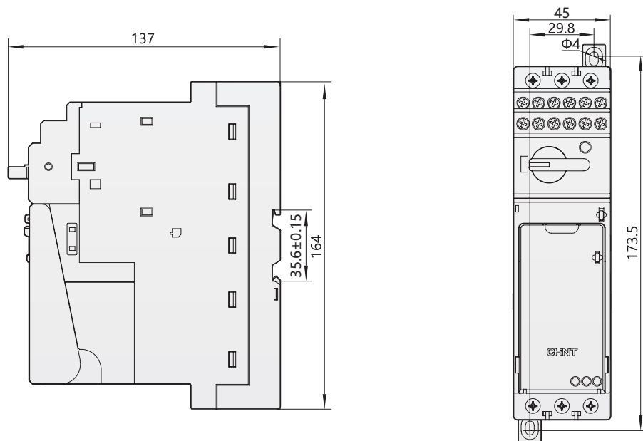
Рис. 5. Внешний вид и установочные размеры NKB8G
