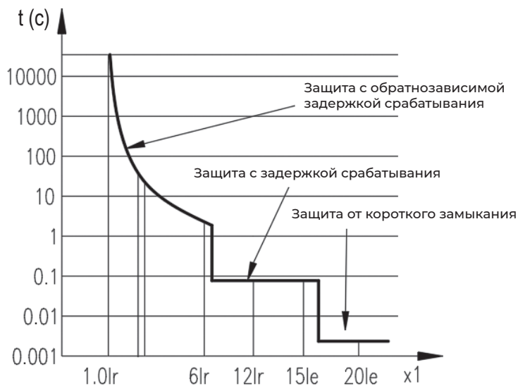
Рис. 1. Время-токовая характеристика
